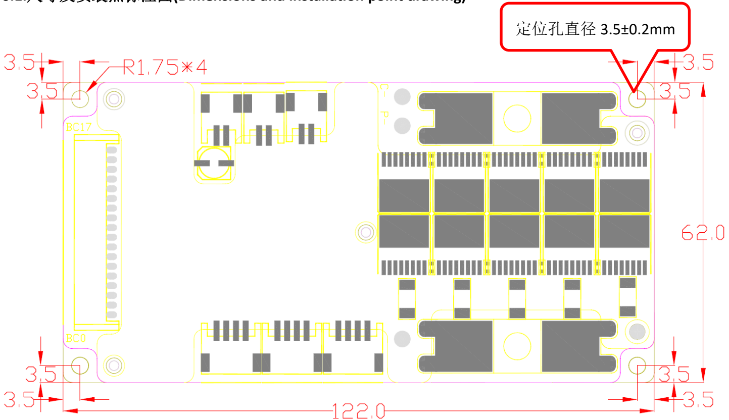
结构尺寸图（单位：毫米） Figure of structure size(unit:mm)
